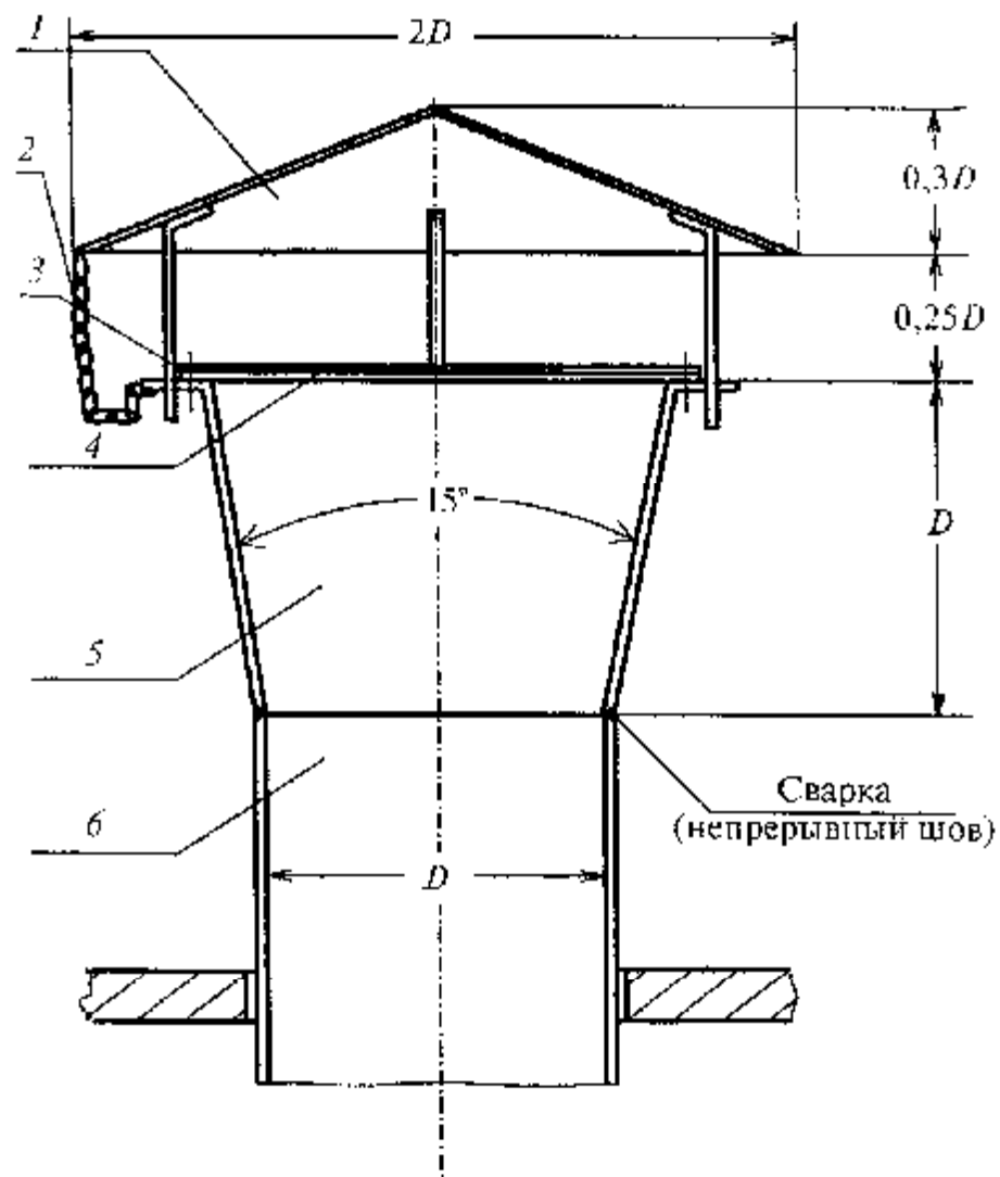
Рис. 7. Конструктивная схема взрывозащитного устройства с диффузором на срезе короткого вертикального патрубка:
