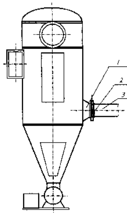
Рис. 18. Схема расположения взрыворазрядного устройства на фильтр-циклоне:
