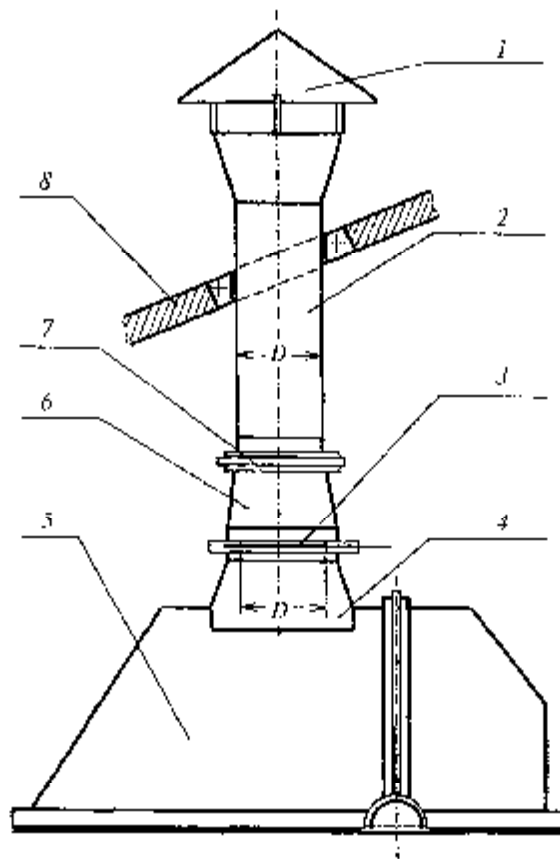
Рис. 9. Схема расположения на головке норы взрыворазрядного устройства шieberного типа:
