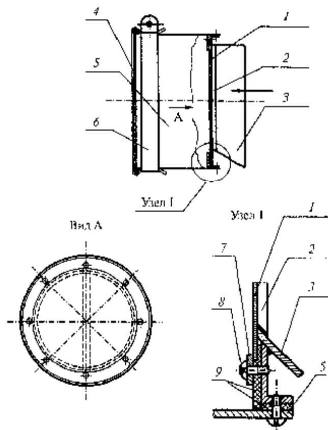
Рис. 5. Конструктивная схема взрыворазрядного устройства с выщелкивающейся мембраной:
