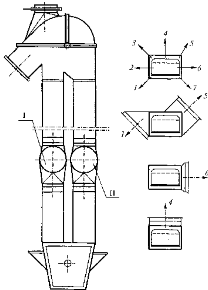
Рис. 14. Возможные варианты расположения взрыворазрядных устройств на норийных трубах: 1, 2, 3 ... — возможные направления оси взрыворазрядного устройства
