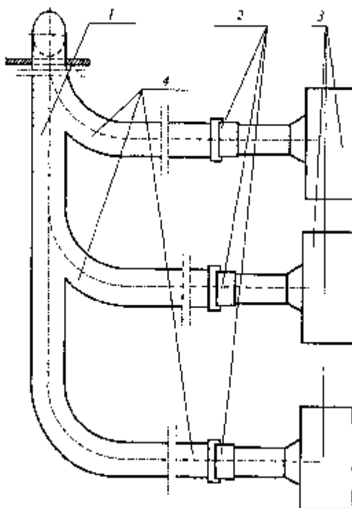
Рис. 20. Схема установки на группе оборудования комбинированных взрыворазрядных устройств, объединенных коллектором:
