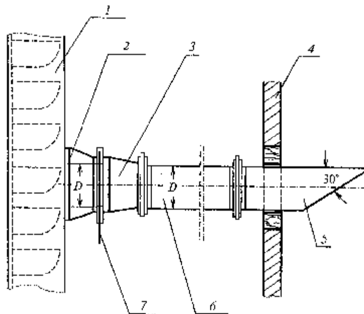
Рис. 13. Схема расположения на норийной трубе взрыворазрядного устройства шиберного типа:
