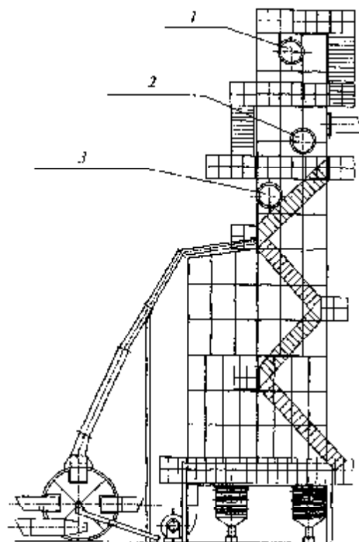
Рис. 19. Схема расположения взрыворазрядных устройств на зерносушилке РД-2(25-70):
