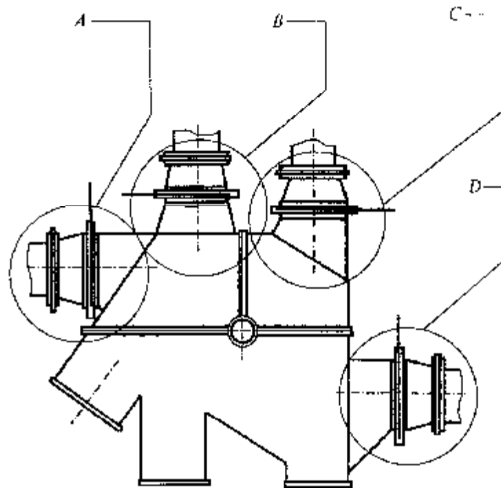
Рис. 10. Возможные варианты расположения взрыворазрядных устройств на головке нории с гравитационной разгрузкой:
