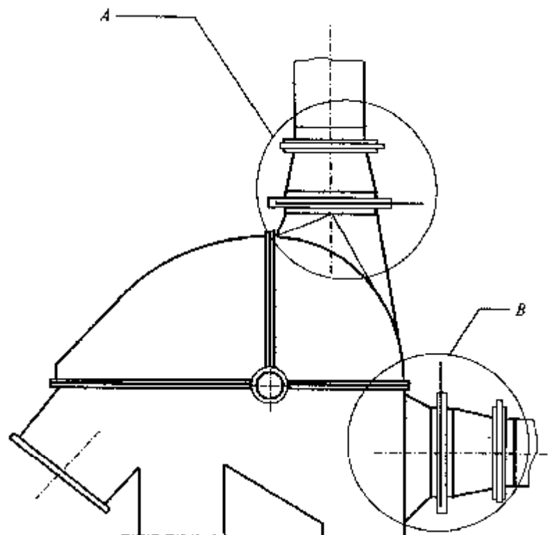
Рис. 11. Возможные варианты расположения взрыворазрядных устройств на головке нории с центробежно-гравитационной разгрузкой:
