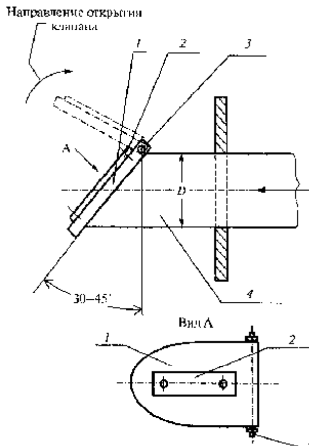
Рис. 4. Конструктивная схема взрыворазрядного устройства с откидным клапаном и горизонтальным отводящим трубопроводом:
