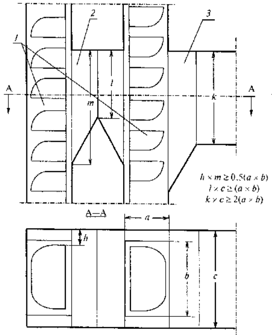
Рис. 15. Схема объединения норийных труб для установки общего взрыворазрядного устройства (1 вариант):
