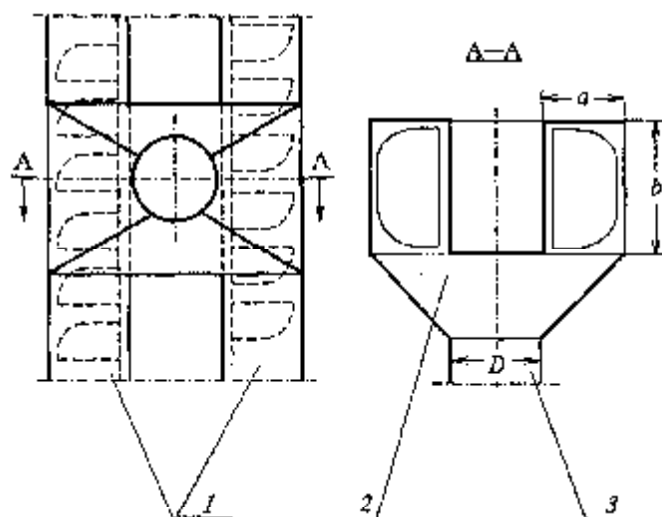
Рис. 16. Схема объединения норийных труб для установки общего взрыворазрядного устройства (II вариант):
