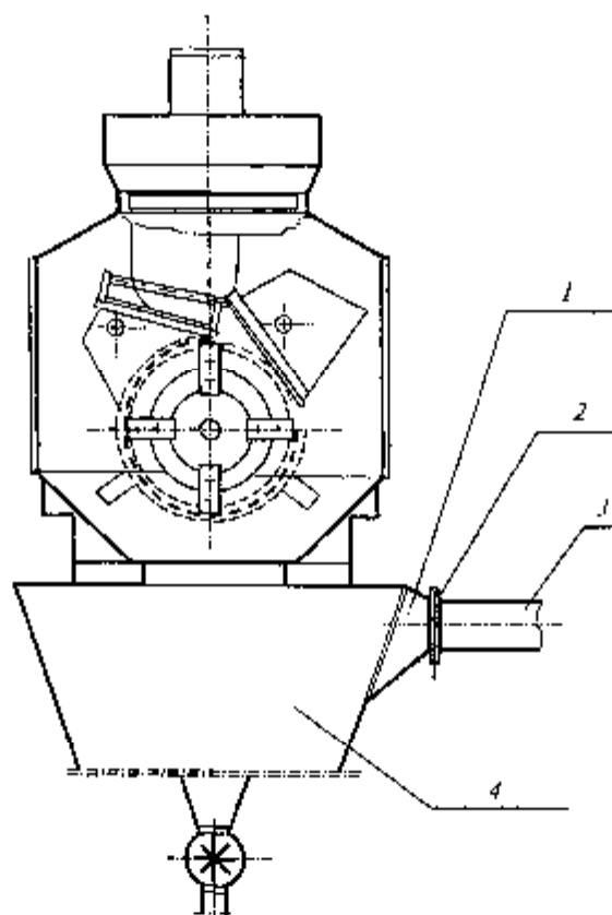
Рис. 17. Схема расположения взрыворазрядного устройства на подробильном бункере:
